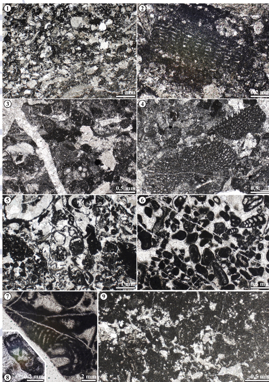
Slika 1: Mikrofacies in fosili vzorčenih artefaktov. 1: Bioklastični intraklastični packstone. Puščica kaže na fragment školjke. Artefakt 510:LJU;0048569. 2: Fragment nedoločene foraminifere. Artefakt 510:LJU;0048569. 3: Bioklastični intraklastični packstone. Artefakt 510:LJU;0055255. 4: Foraminifere naddružine Orbitolinoidea (O). Artefakt 510:LJU;0055255. 5: Bioklastični intraklastični grainstone. Puščica kaže na prekristaljeno hišico polža. Artefakt 510:LJU;0060180. 6: Peloidni grainstone. Črna puščica kaže na foraminifero, bela puščica na fragment lupine mehkužca z mikritiziranim robom. Artefakt 510:LJU;0060203. 7: Foraminifera Orbitopsella primaeva Henson. Artefakt 510:LJU;0060203. 8: Foraminifera Everticyclammina praevirguliana Fugagnoli. Artefakt 510:LJU;0060203. 9: Delno spran mudstone z redkimi klasti. Črka P označuje fekalni pelet. Artefakt 510:LJU;0059824.
